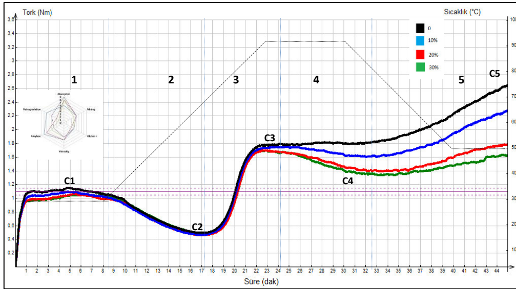
Şekil 2. Farklı oranlarda ince kepek katkılı hamurların miksolab eğrileri
