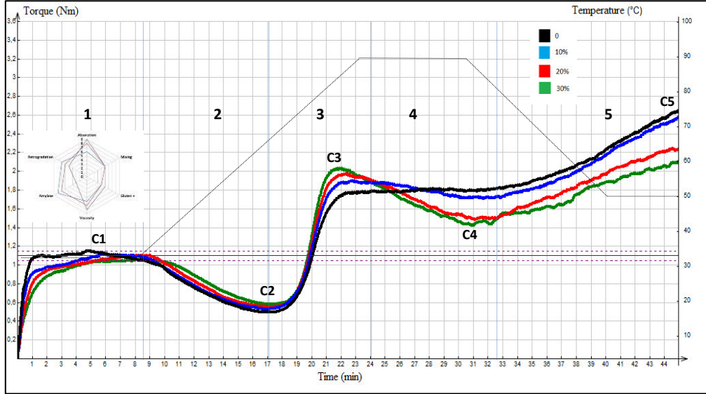
Şekil 1. Farklı oranlarda kaba kepek katkılı hamurların miksolab eğrileri
